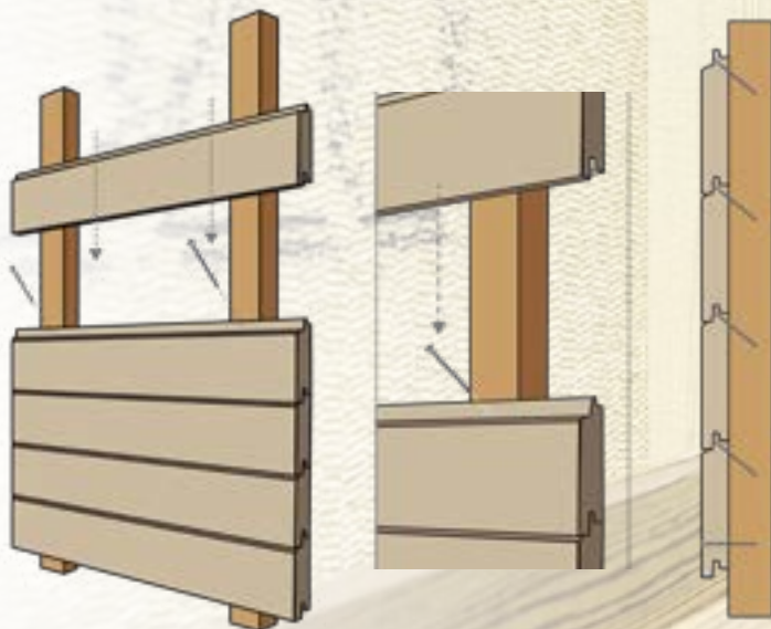
EXEMPLE D'UNE POSE À EMBOÎTEMENT Bardage avec recouvrement
